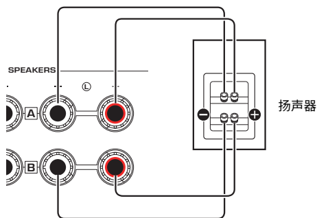
后面板
