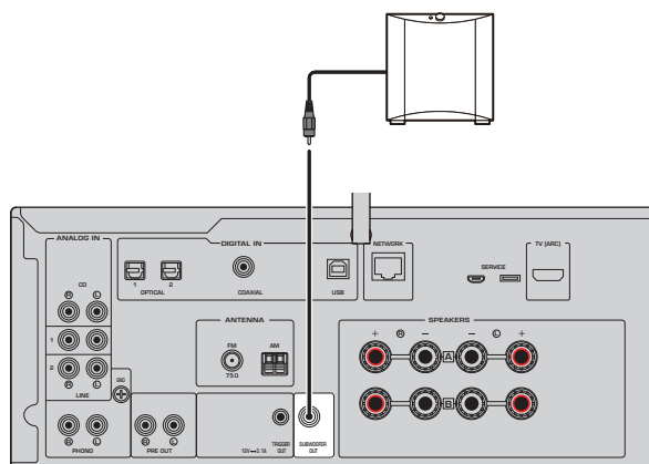
后面板
